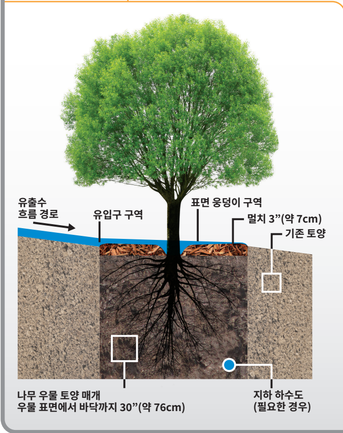
나무 우물 (단면도)
